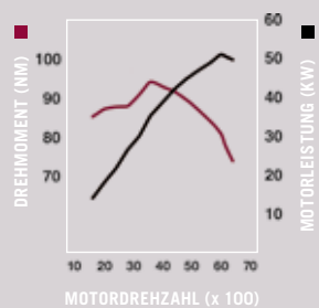
1,0-Liter-Motor
